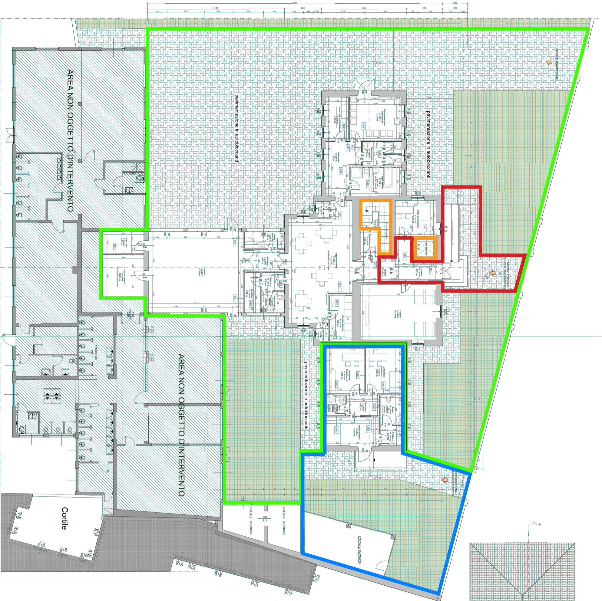
PROGETTO_PIANO TERRA
